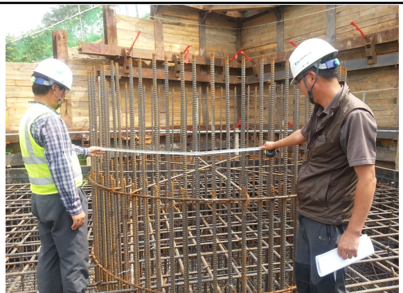
P6 기초 시공 상태 검측
