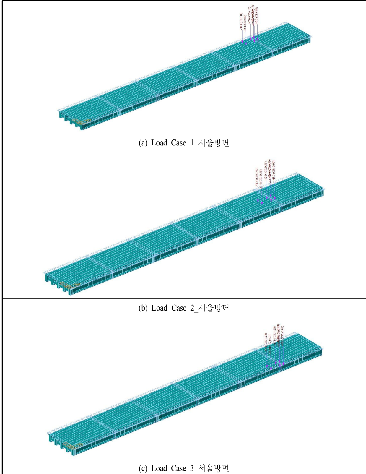
<그림 4.4.2> 신평2교(서울방면) Load Case별 하중재하도
