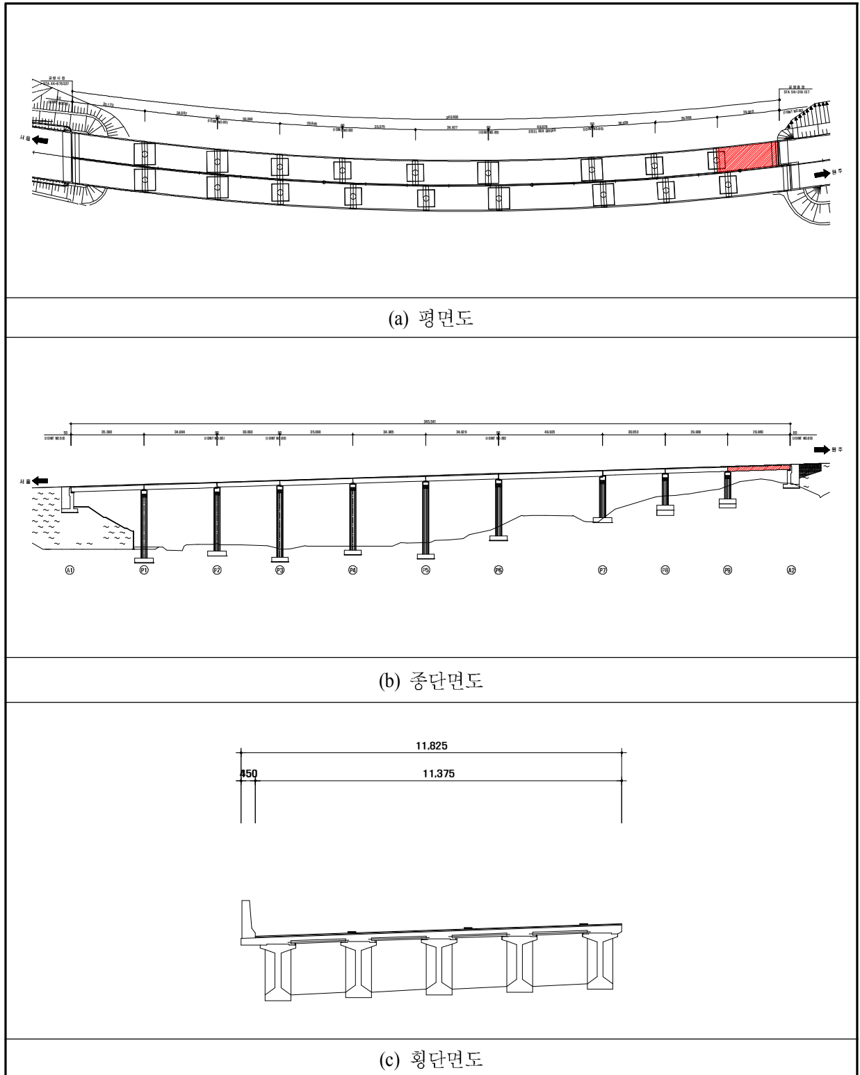
<그림 4.3.1> 신평2교 (서울방향) 평면도, 종단면도 및 횡단면도
