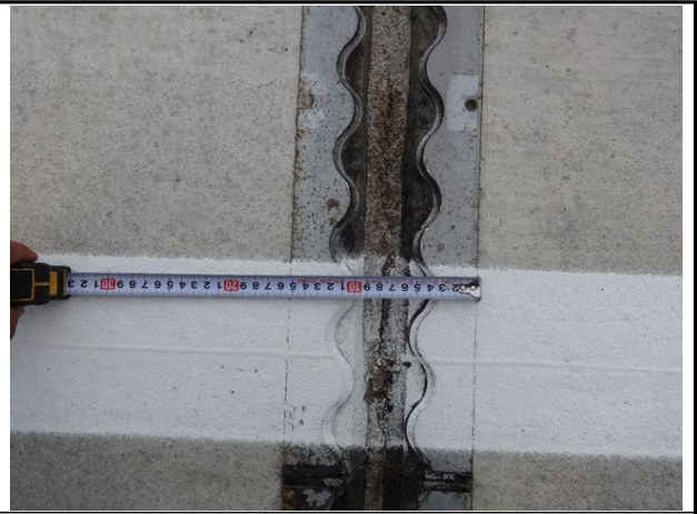
신축이음 A1 유간 측정
