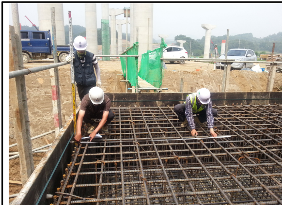
P6 기초 철근 배근 간격 측정
