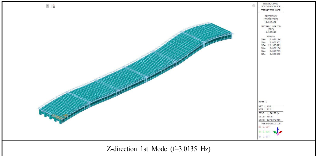
<그림 4.4.3> 신평2교(서울방면) 고유치 해석
